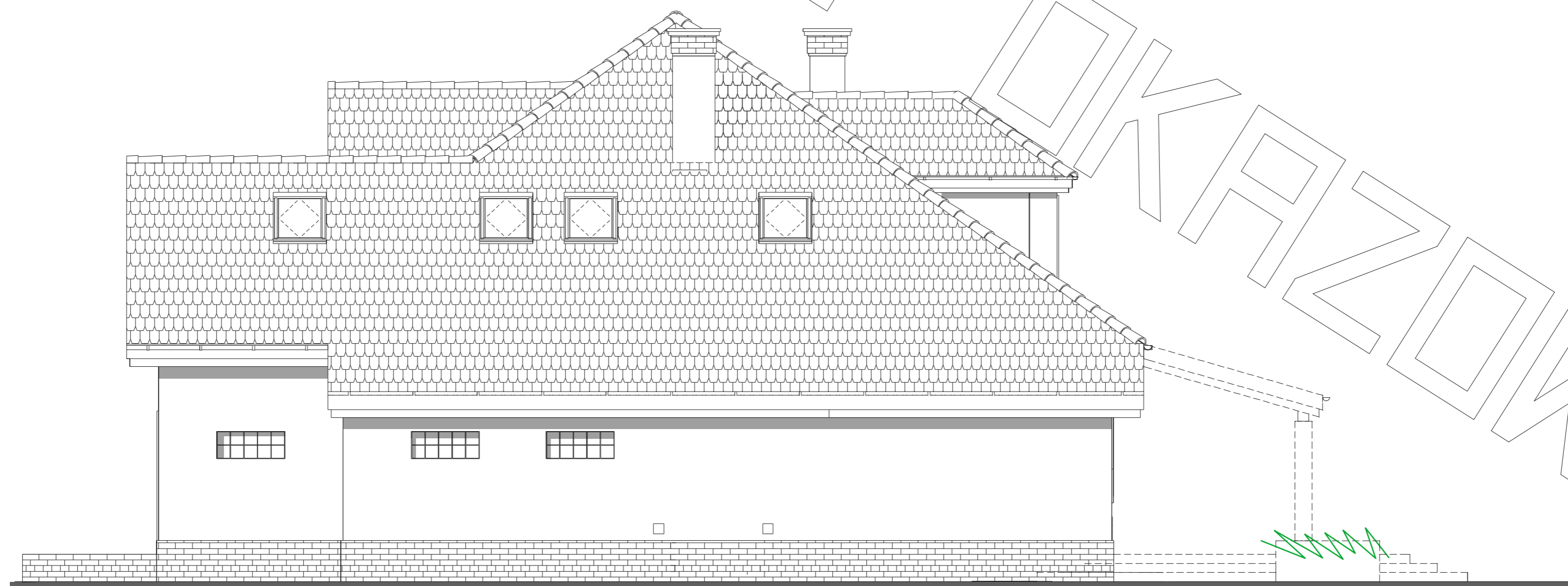
elewacja boczna
