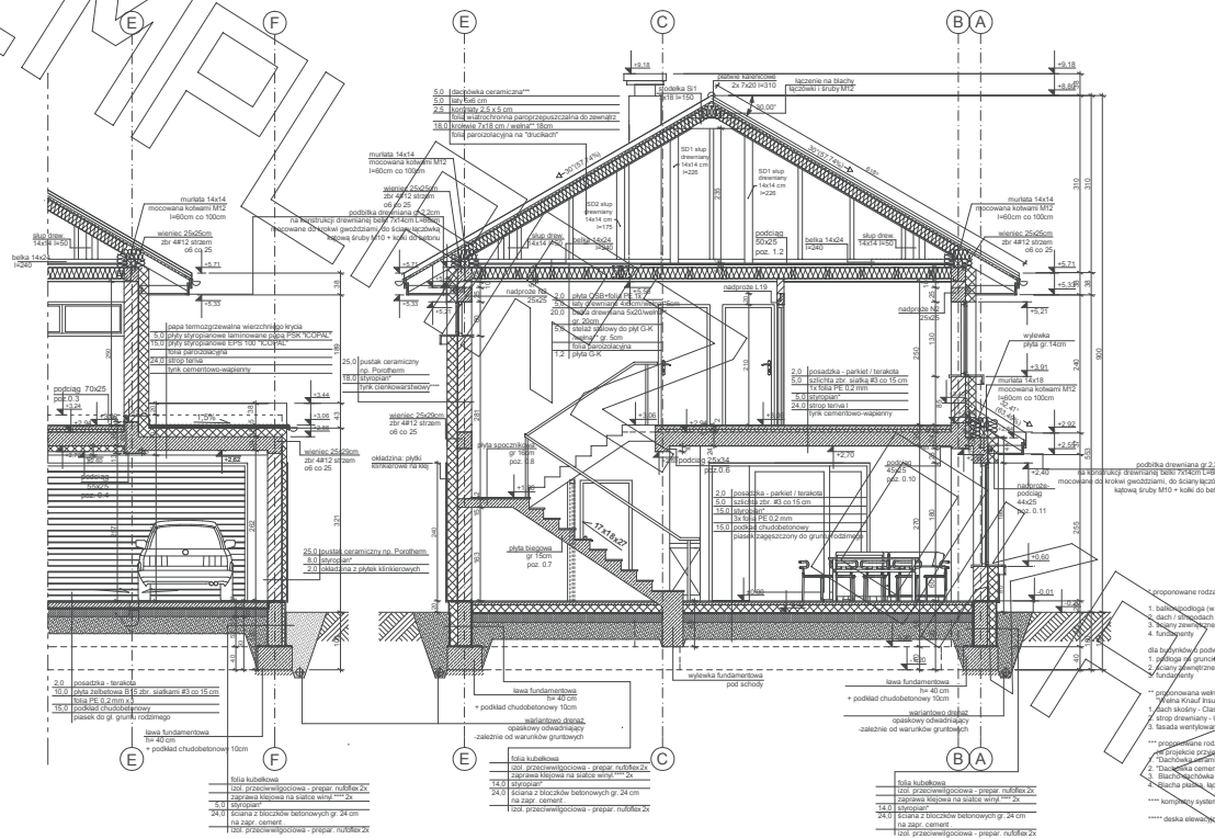
Przekrój A'-A'
