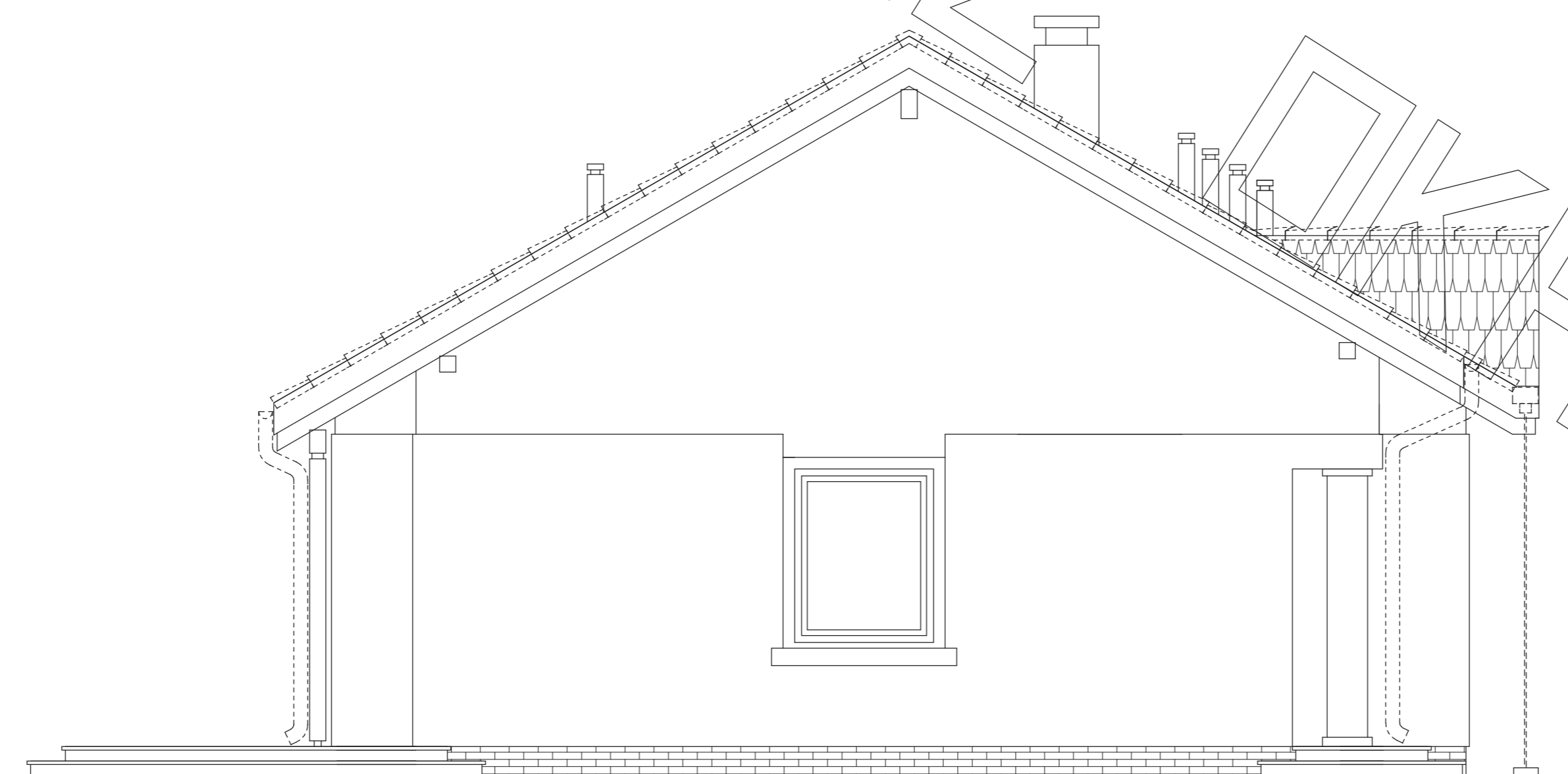
elewacja boczna
